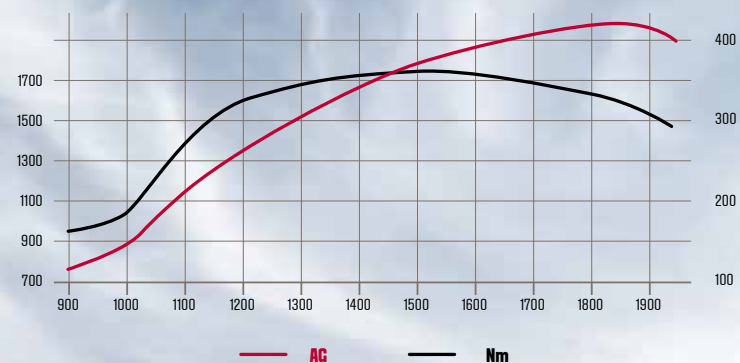
SUKIMO MOMENTAS (Nm), S396 IR S416
